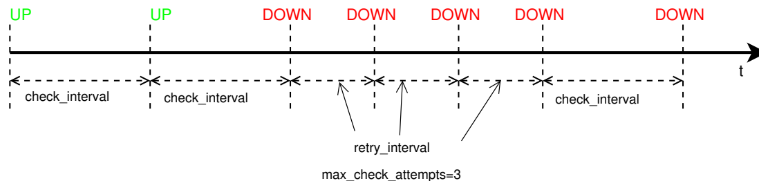
Figure 8: Esquema temporal de parámetros de disponibilidad en Nagios
