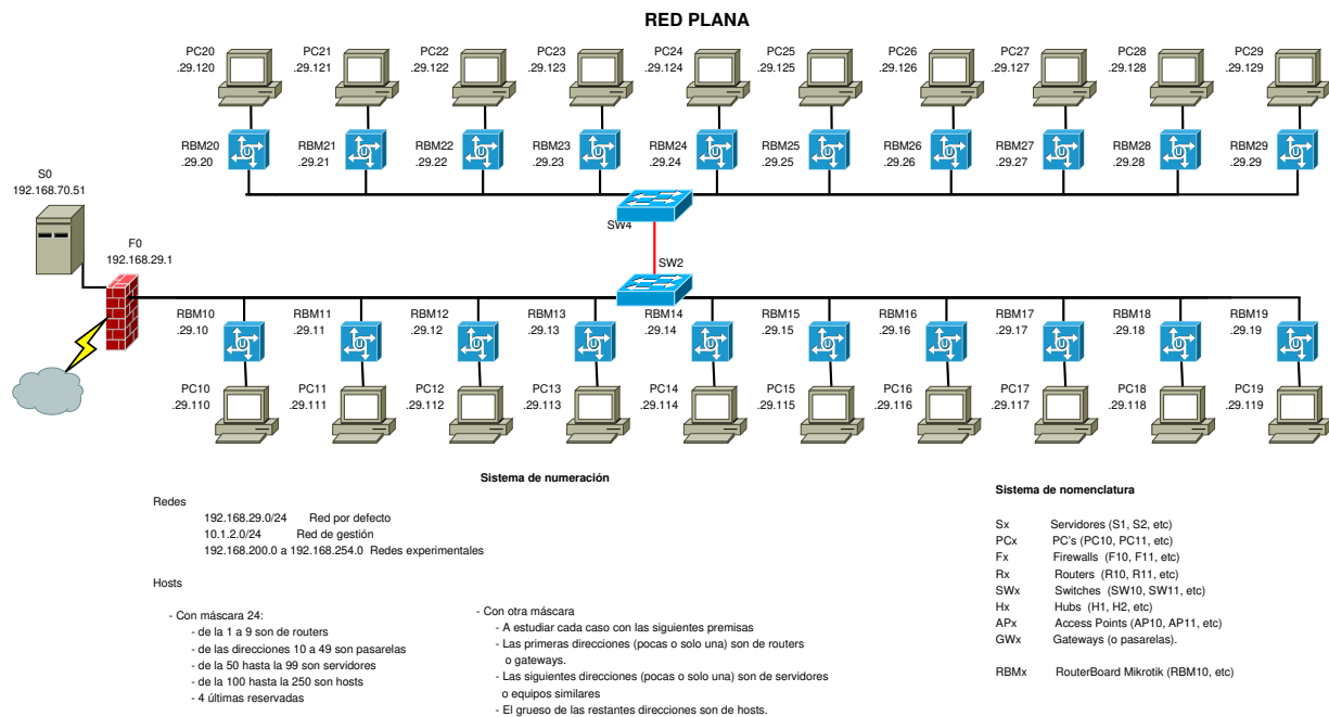
Figure 1: Red de monitorización del laboratorio
