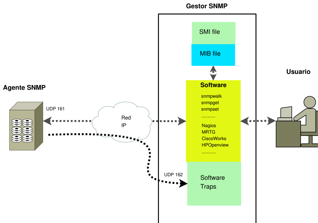
Figure 2: Topología básica SNMP
